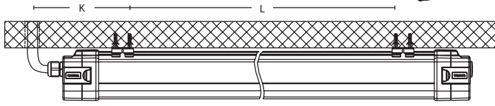
Bohrschablonen für Decken- oder Wandbefestigung
