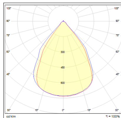
Lichtverteilungskurve MODUL 100 1200mm
