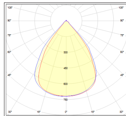
Lichtverteilungskurve MODUL 200 1500mm
