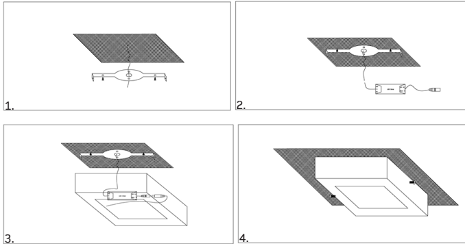
Abb. 3: ASTERION G2 quadratisch Installationsreihenfolge
