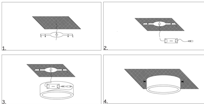
Abb. 4: ASTERION G2 rund Installationsreihenfolge
