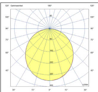
Lichtverteilungskurve BOLT R1200 105°
