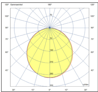
Lichtverteilungskurve BOLT R900 down 105° up Ambiente
