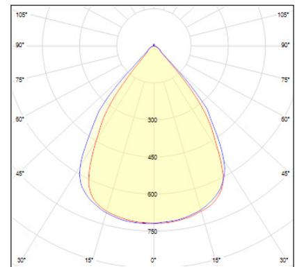
Lichtverteilungskurve MODUL 100 1500mm
