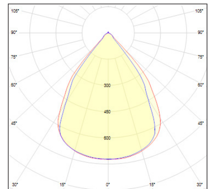
Lichtverteilungskurve MODUL 600 PRO zweilampig
