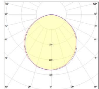
Lichtverteilungskurve WEGA ON-TOP 1.547mm
