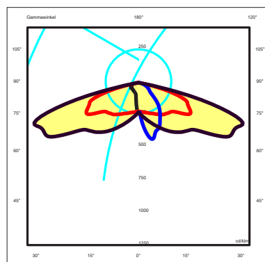
Lichtverteilungskurve STREET PRO L5
