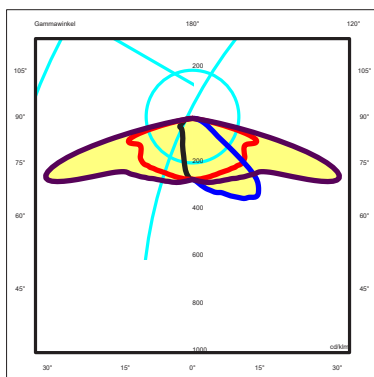
Lichtverteilungskurve STREET PRO L1
