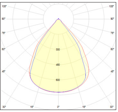
Lichtverteilungskurve MODUL 625 zweilampig
