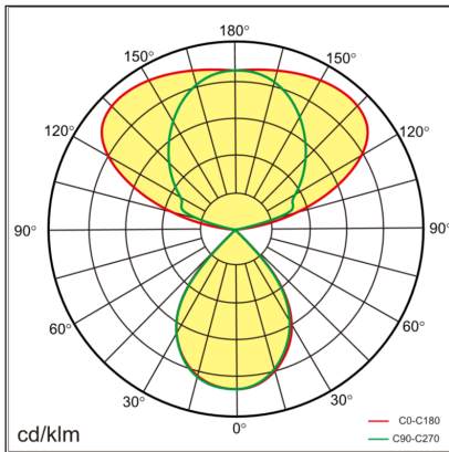
Lichtverteilungskurve SECRET SL-U 75° direkt 150° indirekt
