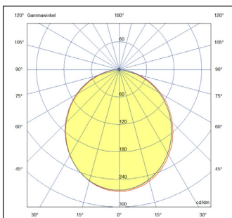
Lichtverteilungskurve BOLT R380 down 105° up Ambiente
